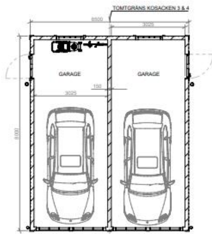
SEKTION A-A
