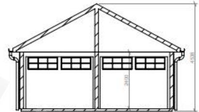
SEKTION B-B
