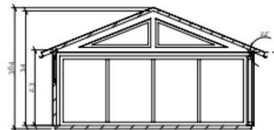
SEKTION D-D
